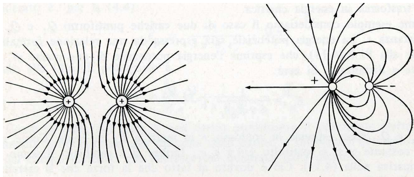
+2q, -q
